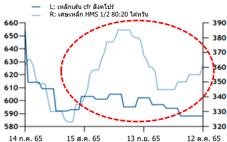
เศษเหล็กเอเชีย vs เหล็กเส้น
